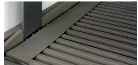
Laufstege auf Trapezblech für bessere Begehbarkeit
